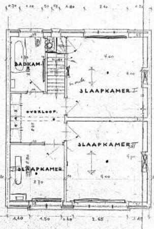
PLAN DER VERDIEPING.
