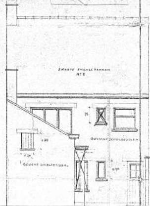
ACHTERGEVEL.
