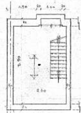
KELDERPLAN.
