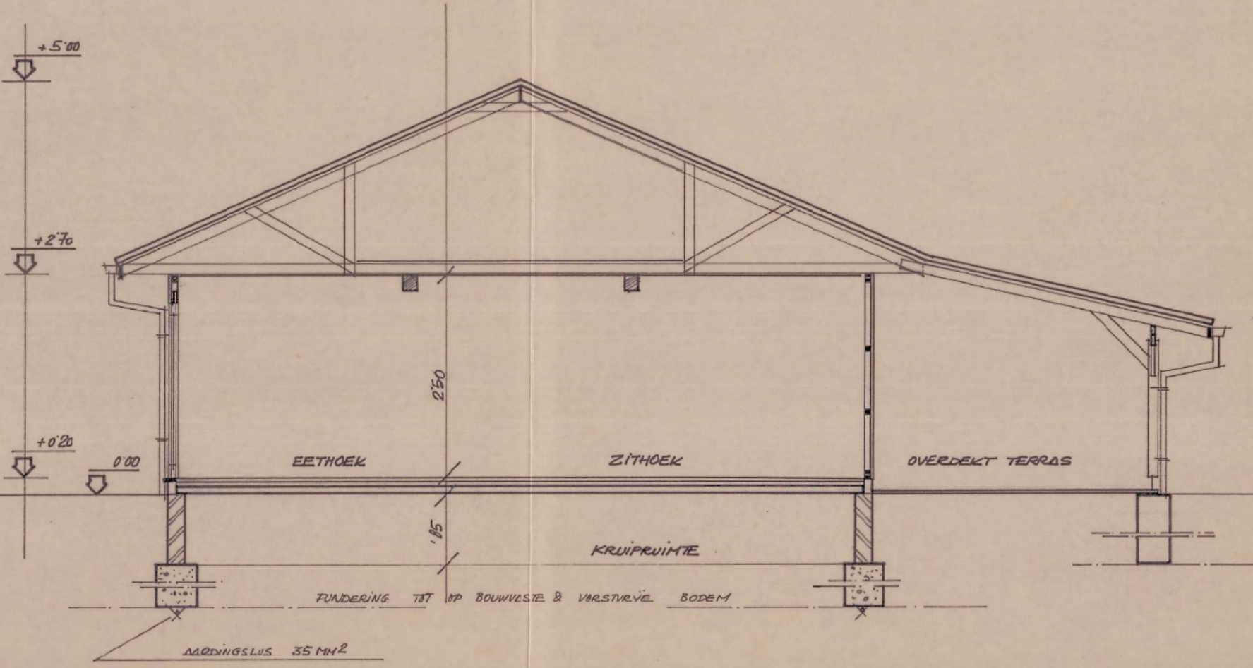
doorsnede
