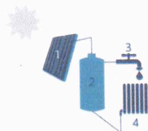
1. Zonnecollector | 2. Opslagvat zonneboiler | 3. Sanitair warm water | 4. Aardwarmte voor ruimteverwarming (optioneel)
